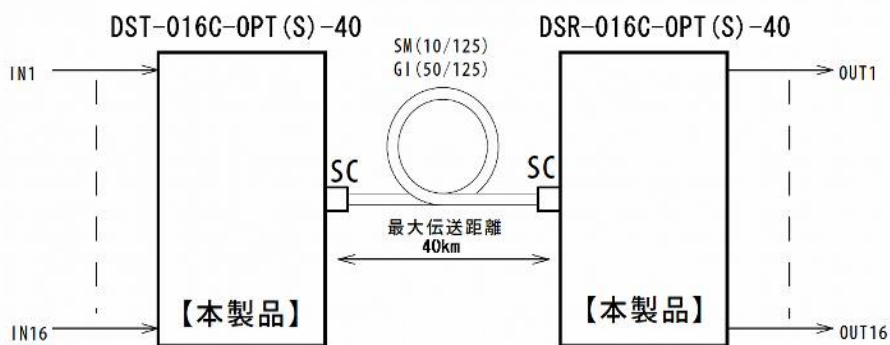
接続構成
